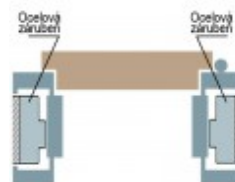
Renovierungszarge
