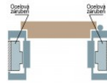
Renovierungszarge
