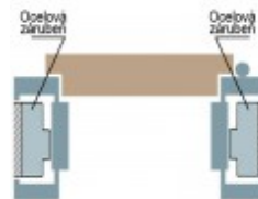
Renovierungszarge
