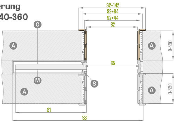
Auf dem Bild schematische Darstellung der beidseitigen Einmauerung ZN1 + ZN1.
